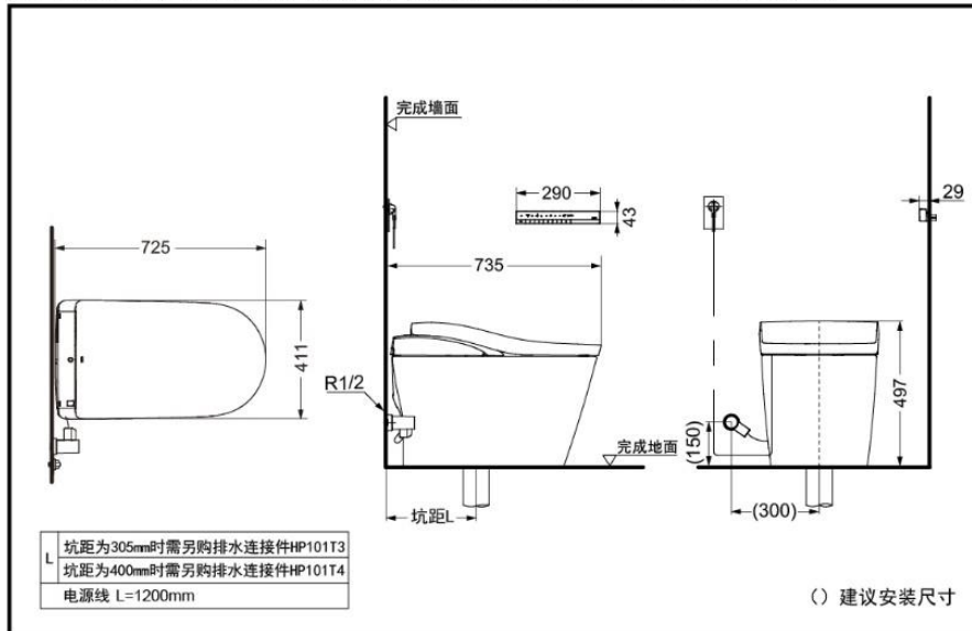
CES8G220GCN · NEOREST One-piece Toilet
