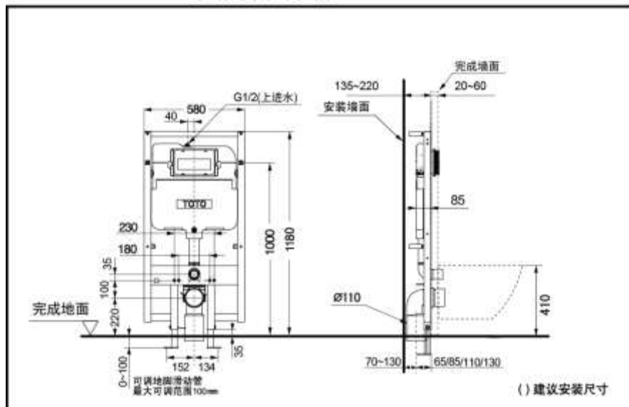
WH173B-553B 手动隐藏式水箱
