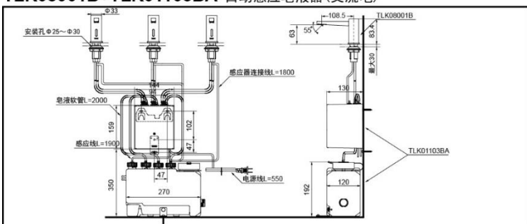
TLK08001B+TLK01103BA 自动感应皂液器 (交流电)
