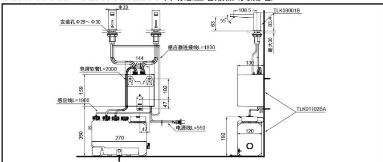
TLK08001B+TLK01102BA 自动感应皂液器 (交流电)
