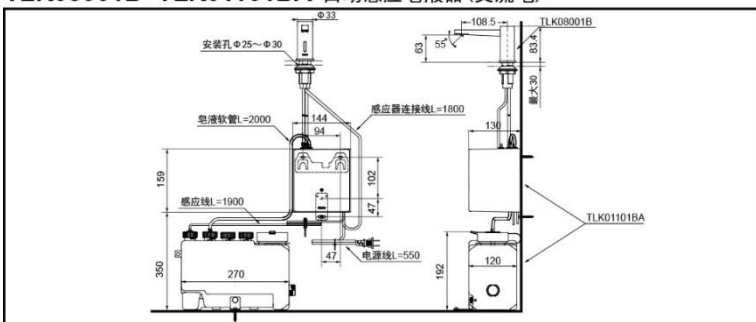
TLK08001B+TLK01101BA 自动感应皂液器 (交流电)
