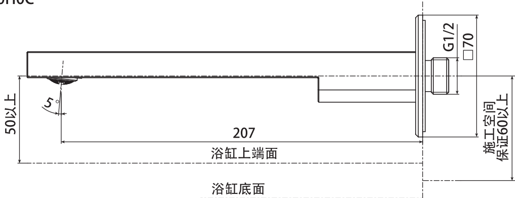
浴用吐水口 TBG160H0C*
