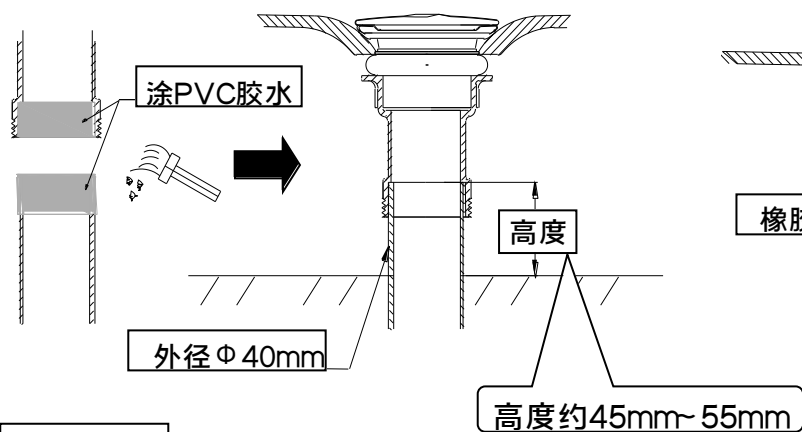
安装示意图
