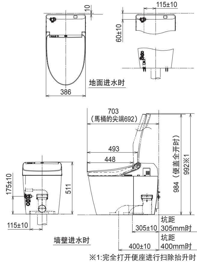
产品安装图（安装完了图）DH型（单位:mm）
