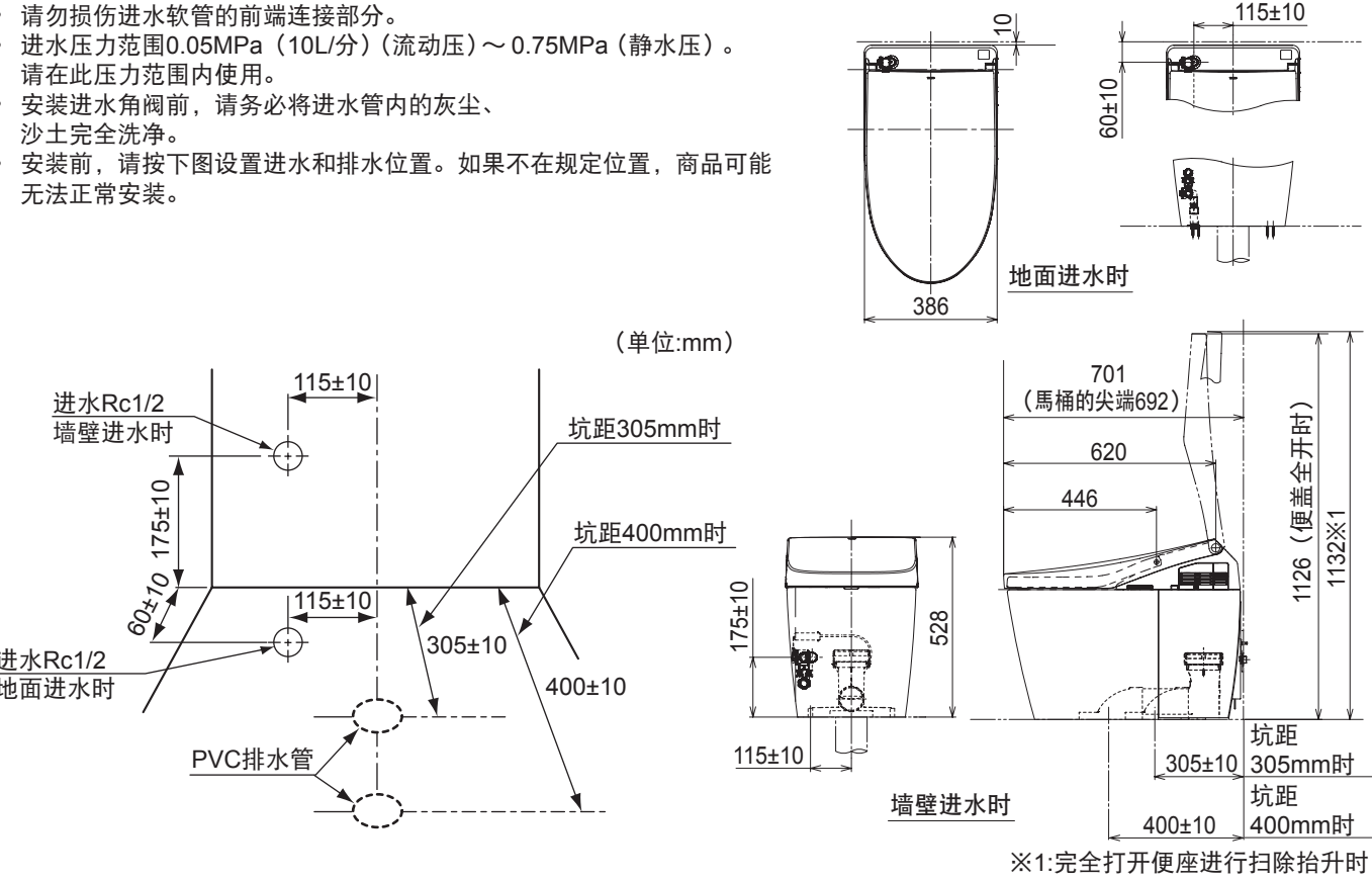
产品安装图（安装完了图）RH型（单位:mm）
