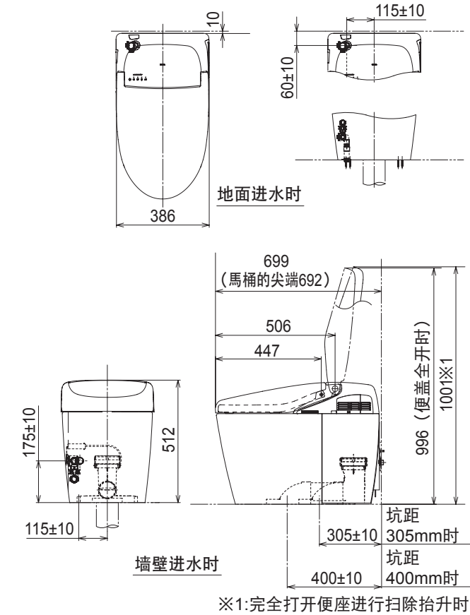
产品安装图（安装完了图）RH型（单位:mm）
