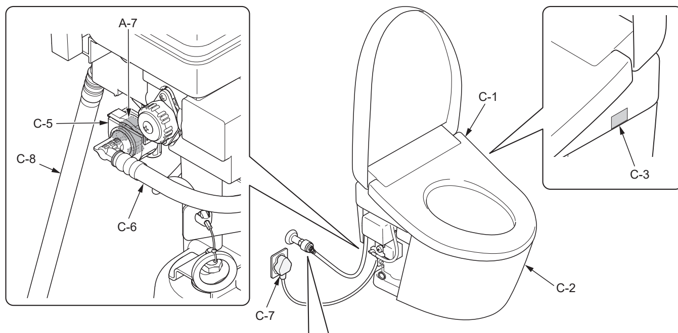
① 墙面进水时
