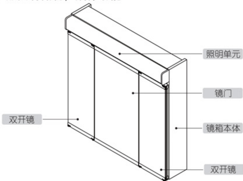
图为LMAW753DR系列、LMAW903DR系列、LMAW1203DR系列
