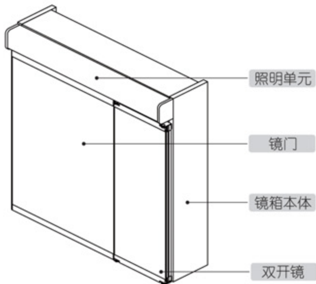
图为LMAW602DR系列、LMAW752DR系列
