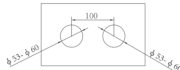
瓷砖开孔尺寸 (单位: mm)
