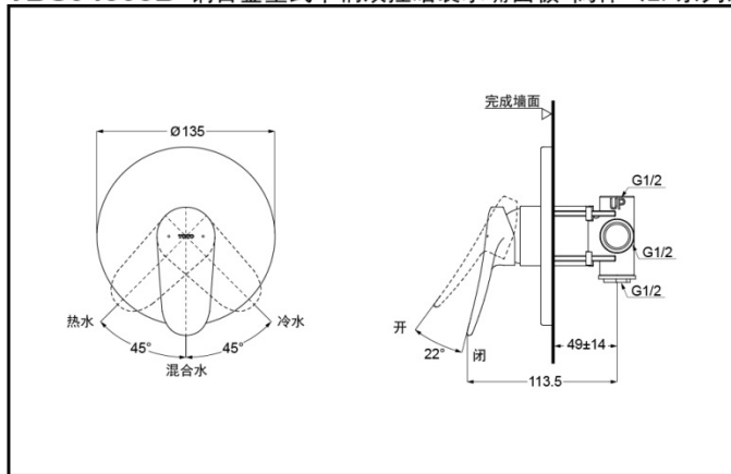
TBS04303B 铜合金壁式单柄双控暗装水嘴面板+阀体（LF系列）
